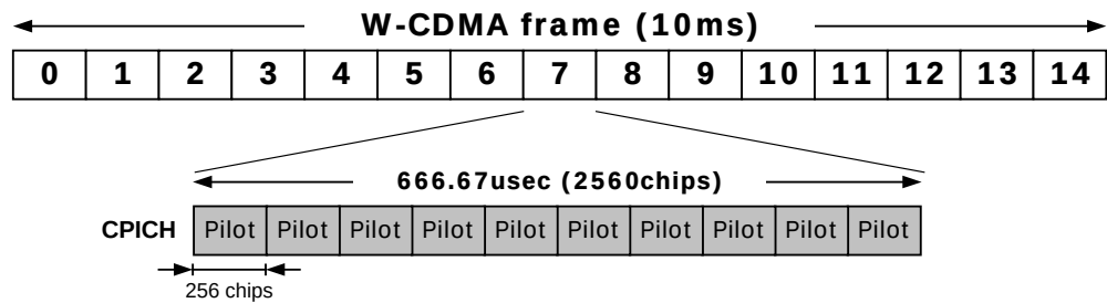
그림4.5.2 공통 파일럿 채널 구조
