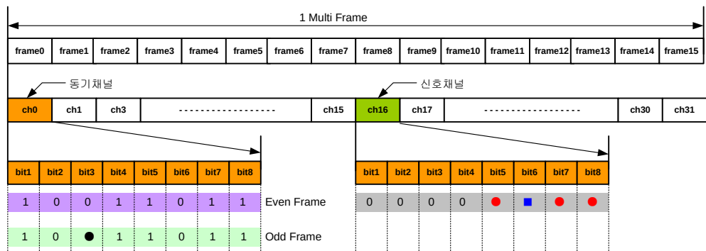
E1 프레임 구조
