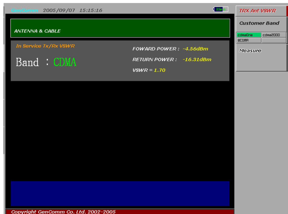
그림6.2.2 TRX Ant VSWR 측정결과 화면
