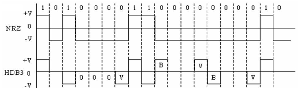
그림8.1.4 HDB3 Line code 방식
