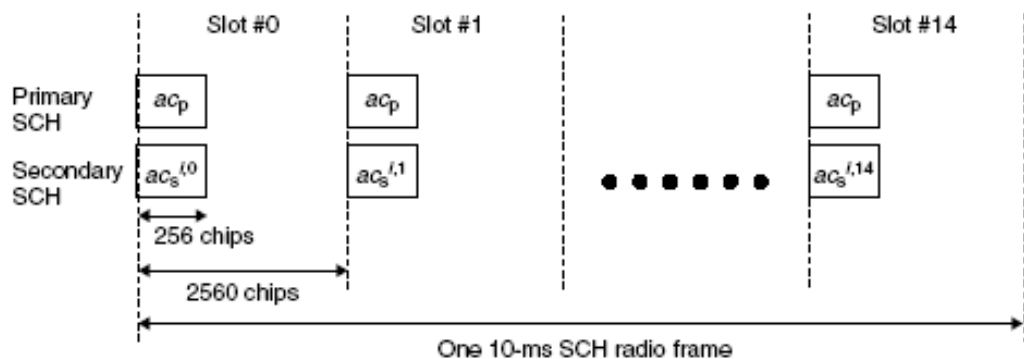
그림4.5.3 동기 채널의 전송 시점과 부호화 코드 부여 방법
